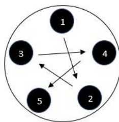
5 Lug Tightening
