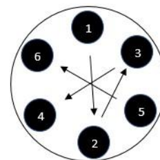
6 Lug Tightening
